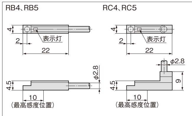
寸法図 (mm)
