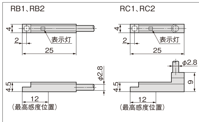
寸法図 (mm)
