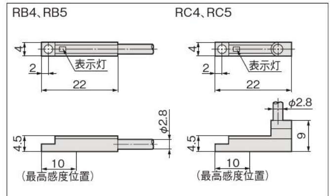
寸法図 (mm)
