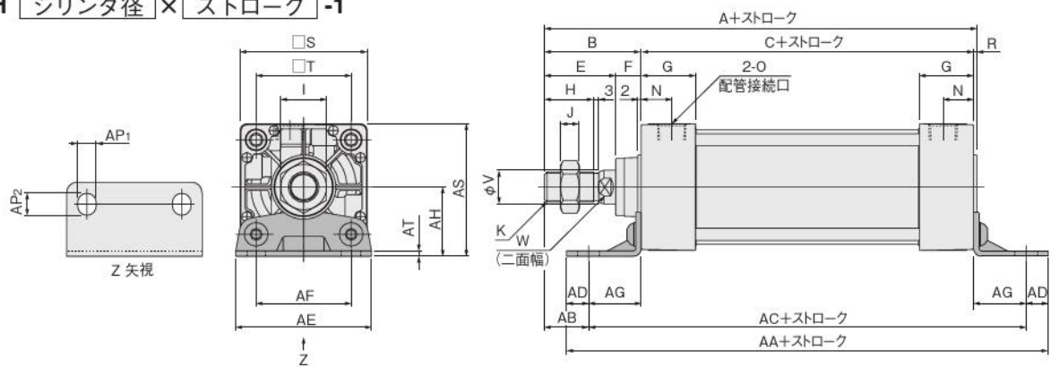
フート形寸法図 (mm)
