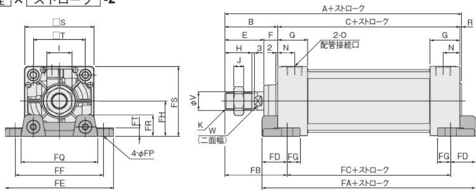
軸直角フート形寸法図 (mm)
