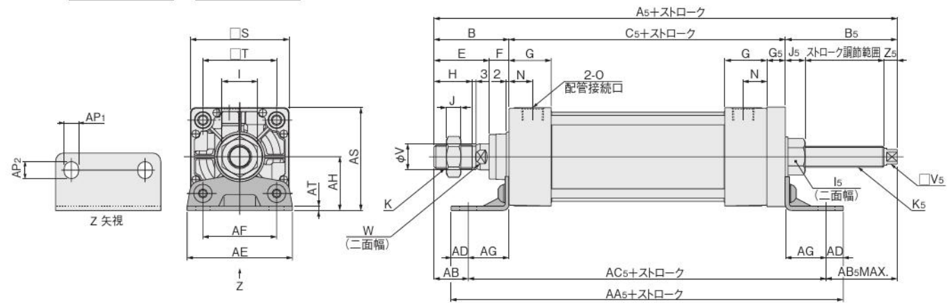
引側ストローク調節フット形寸法図 (mm)
