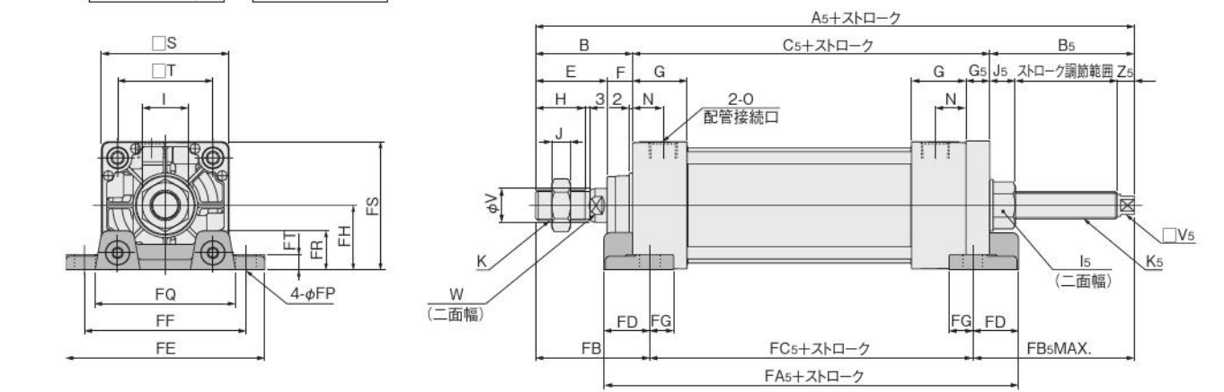
引側ストローク調節軸直角フット形寸法図 (mm)
