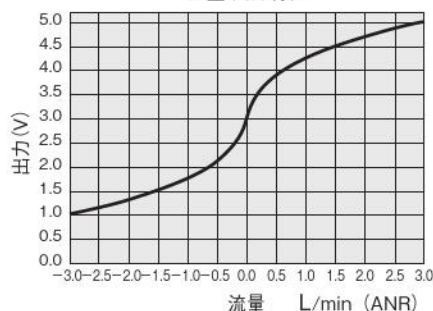
流量-出力特性
