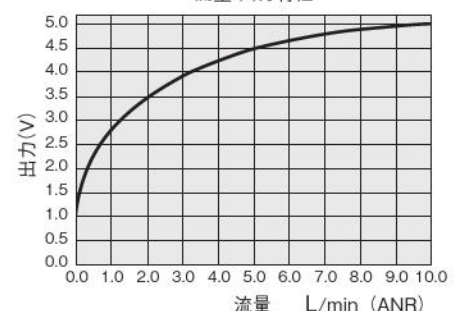
流量-出力特性
