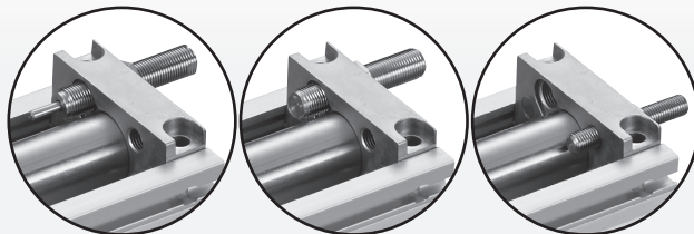
ショックアブソーバ ラバーストoppa メタルストoppa
