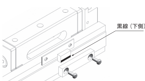
センサマグネットの取付向き
