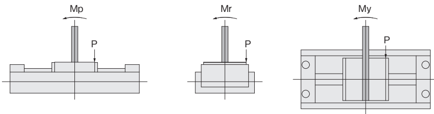
ピッチング方向モーメント ( M_p )
