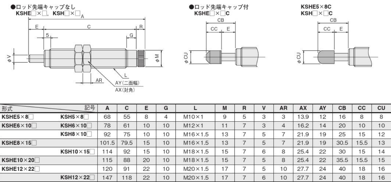
取付金具の寸法図 (mm)
