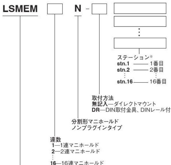
エジェクタマニホールド基本形式
