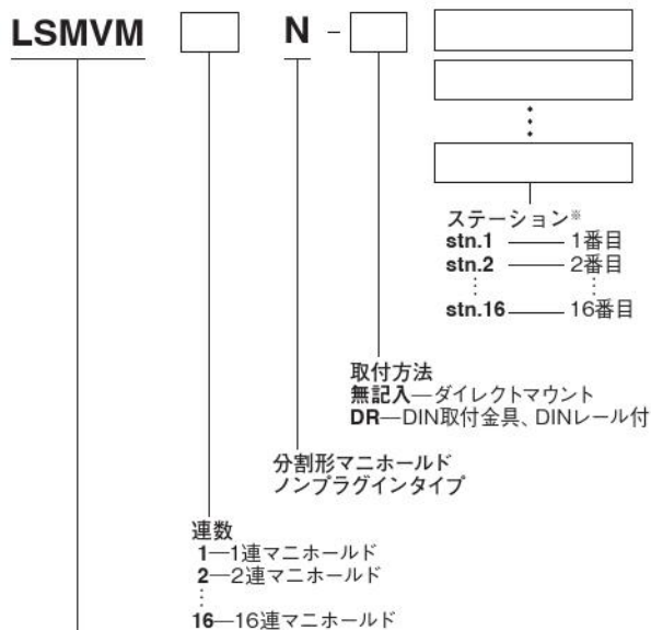
真空バルブユニットマニホールド基本形式
