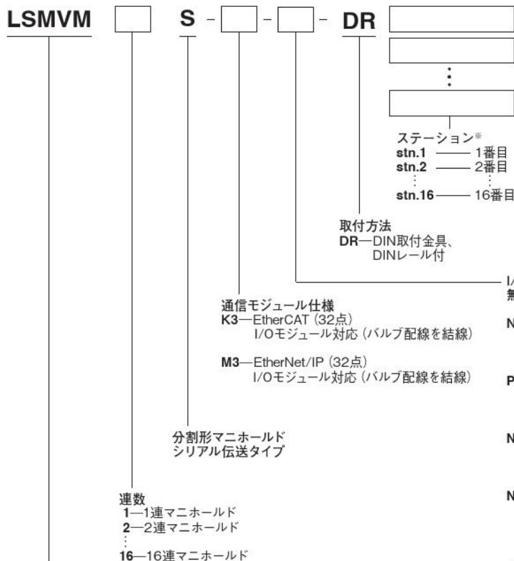
真空バルブユニットマニホールド基本形式
