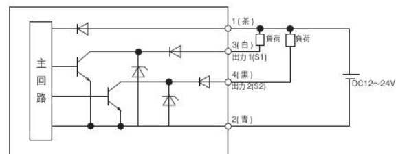
LSMEZ-ND2 (NPN 2点出力タイプ)
