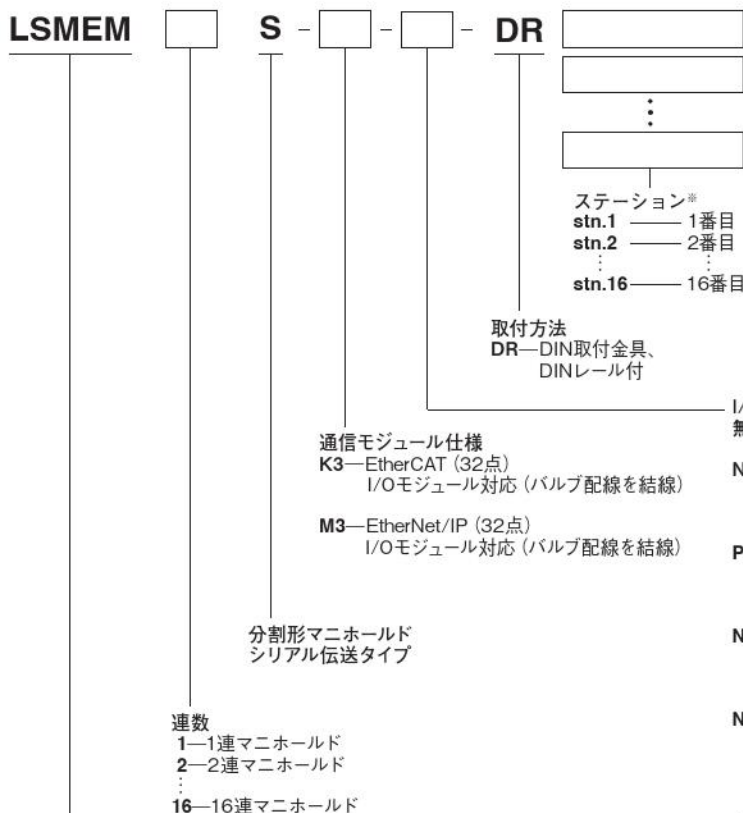
エジェクタマニホールド基本形式
