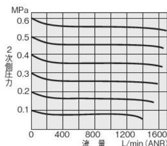
FR300・FR302
