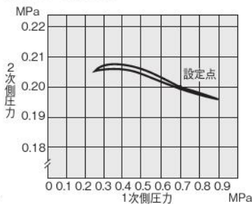
R600・R602
