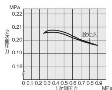
FR600・FR602
