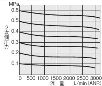
R600・R602
