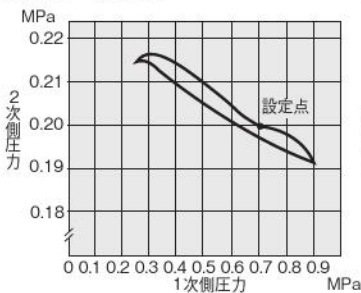
R150・R152
