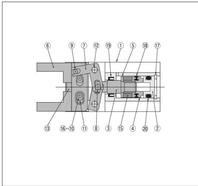
注：図は複動形のレバーが全開の状態です。
