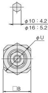
ロッド断面形状
