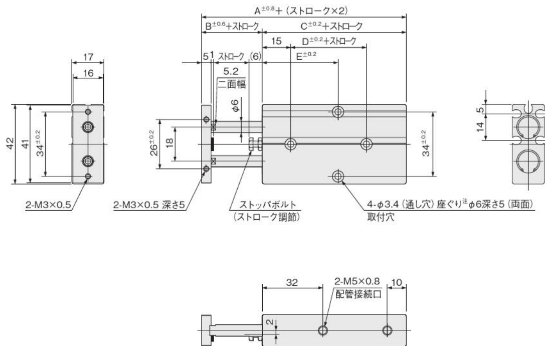
複動ロングブッシュ形寸法図 (mm)
