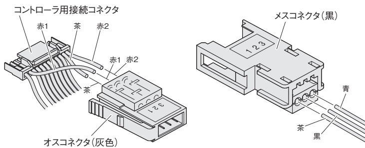
オスコネクタ I/Oコネクタケーブル結線要領
